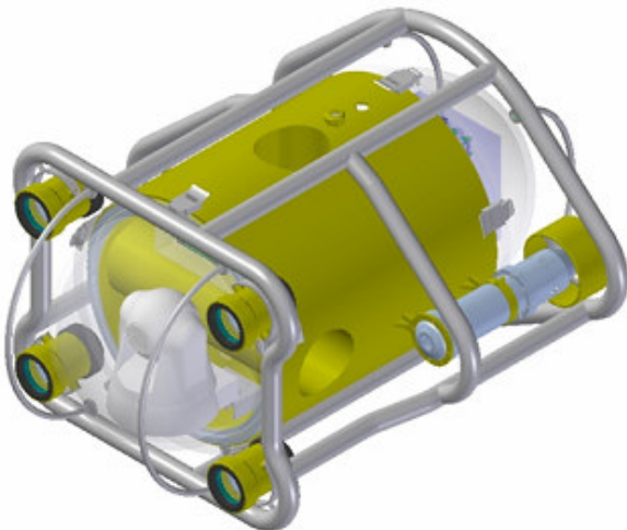
Fig. 2. Diseño básico del vehículo.
